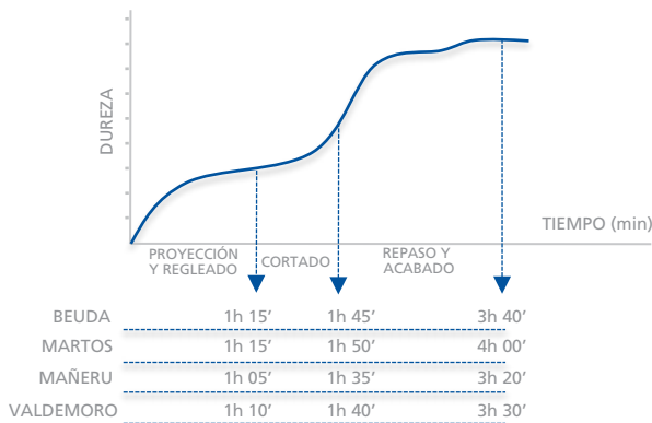
Evolución media de fraguado
