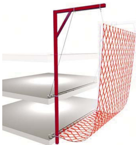
Pescante para Redes Tipo V EN 1263
