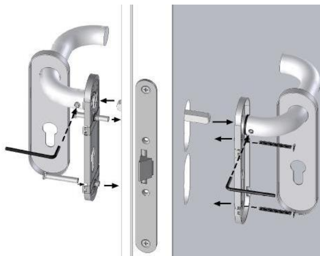
Montaje manilla M0
