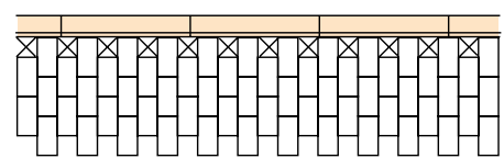
MODELO DE COLOCACIÓN "MATAJUNTA"
