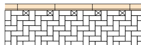
MODELO DE COLOCACIÓN "A 90°"
