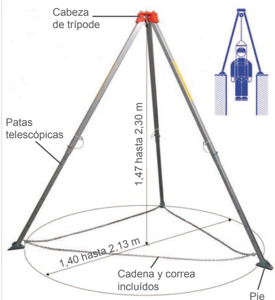
Trípode TRI 9
